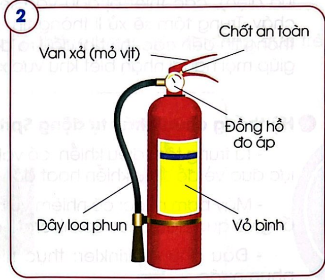
Cấu tạo bình chữa cháy bột
