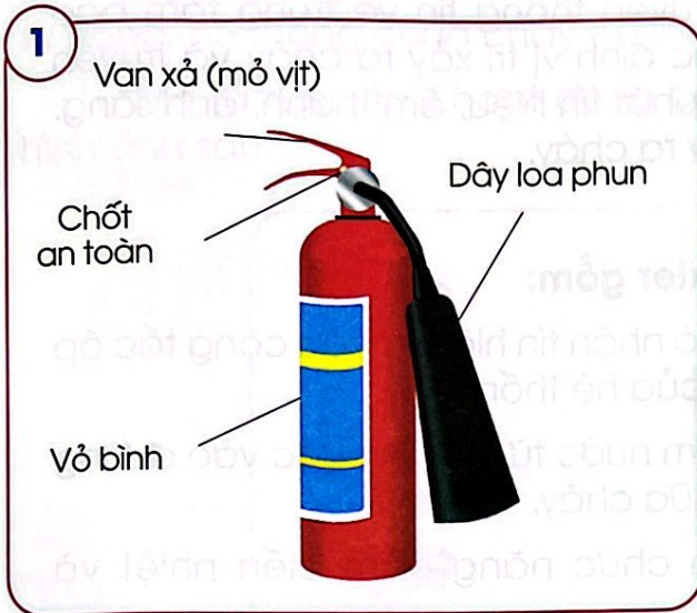
Cấu tạo bình chữa cháy khí \text{CO}_2
